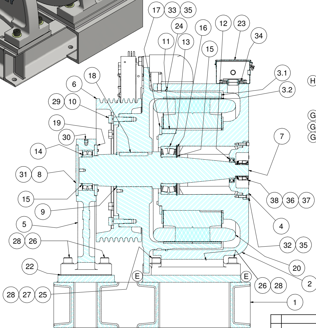
SECTION A-A
